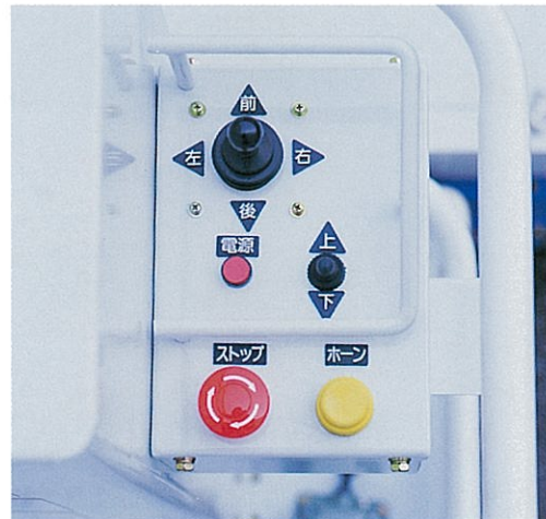
作業床部操作レバー
